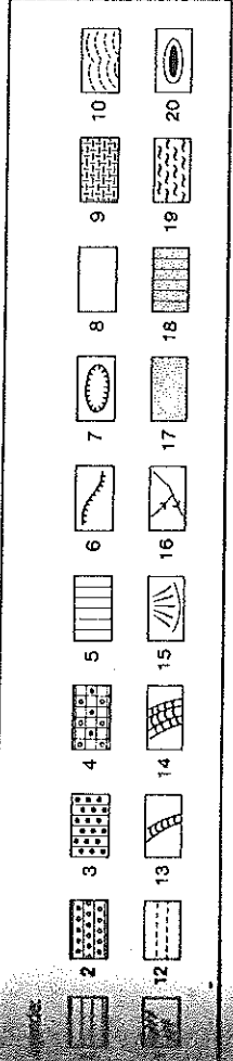
FIGUR 45: 1 = Sanddecke, 2 = rotes Kleinflammenfeld, 3 = schwarzes Kleinflammenfeld, 4 = rote/schwarze Kleinflammen vegetationsgesellschaft, 5 = Hamnada auf Calcrete, 6 = Stufe, 7 = scarp retreat-Pfanne, 8 = Flammenboden, 9 = Barchanfeld, 10 = Dünenfeld (undifferenziert), 11 = Flammenranddünen, 12 = Längsdünen, 13 = Mäldental, 14 = Mäldental mit Hochwasserbett, 15 = Delta, 16 = Talwege in Kerkbultjeif, 17 = Flood plain, auf unreliefte ca-Kruste transgrediert, 18 = Flood plain, auf Kleinflammenfeld transgrediert, 19 = Sandachswenweber, 20 = Inselberge und Rahmenthöhen.
